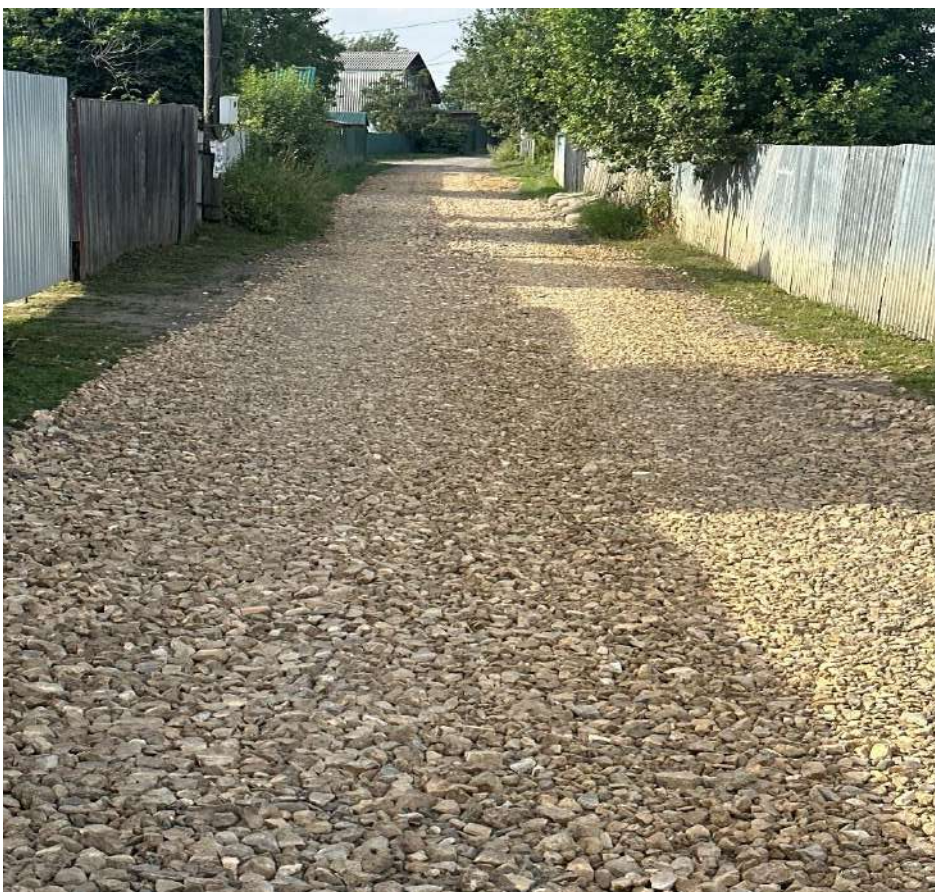
Участок №3806 после отсыпки щебнем фр.40-70 и фр.20-40
